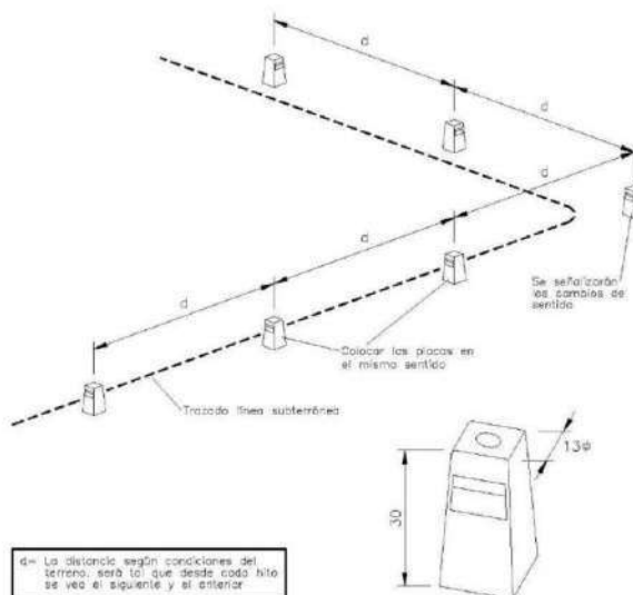
Esquema criterios de ubicación de hitos. Aplicación a hitos rurales.
