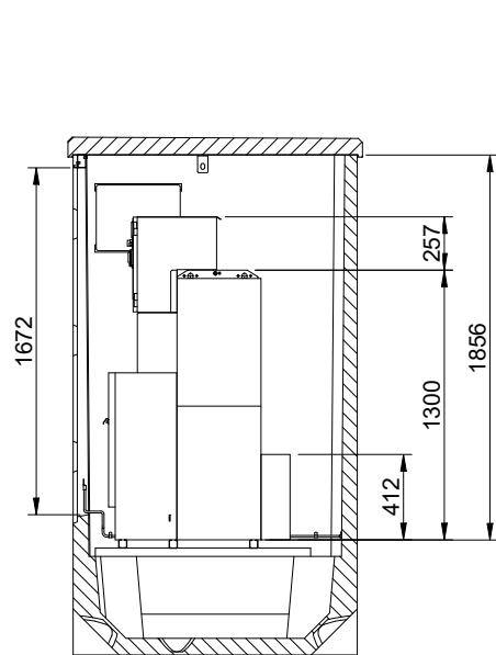
SECCIÓN A-A
