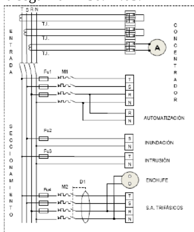
Fig. 3: Esquema del control y alimentación de telegestión
