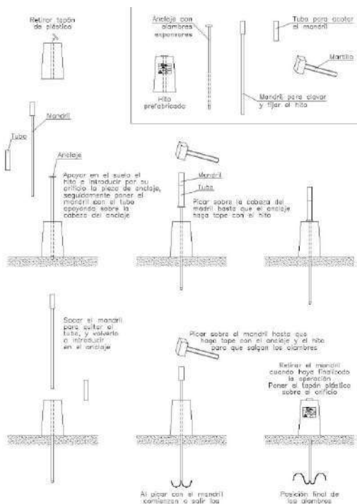
Figura 2: Procedimiento de montaje de hito rural
